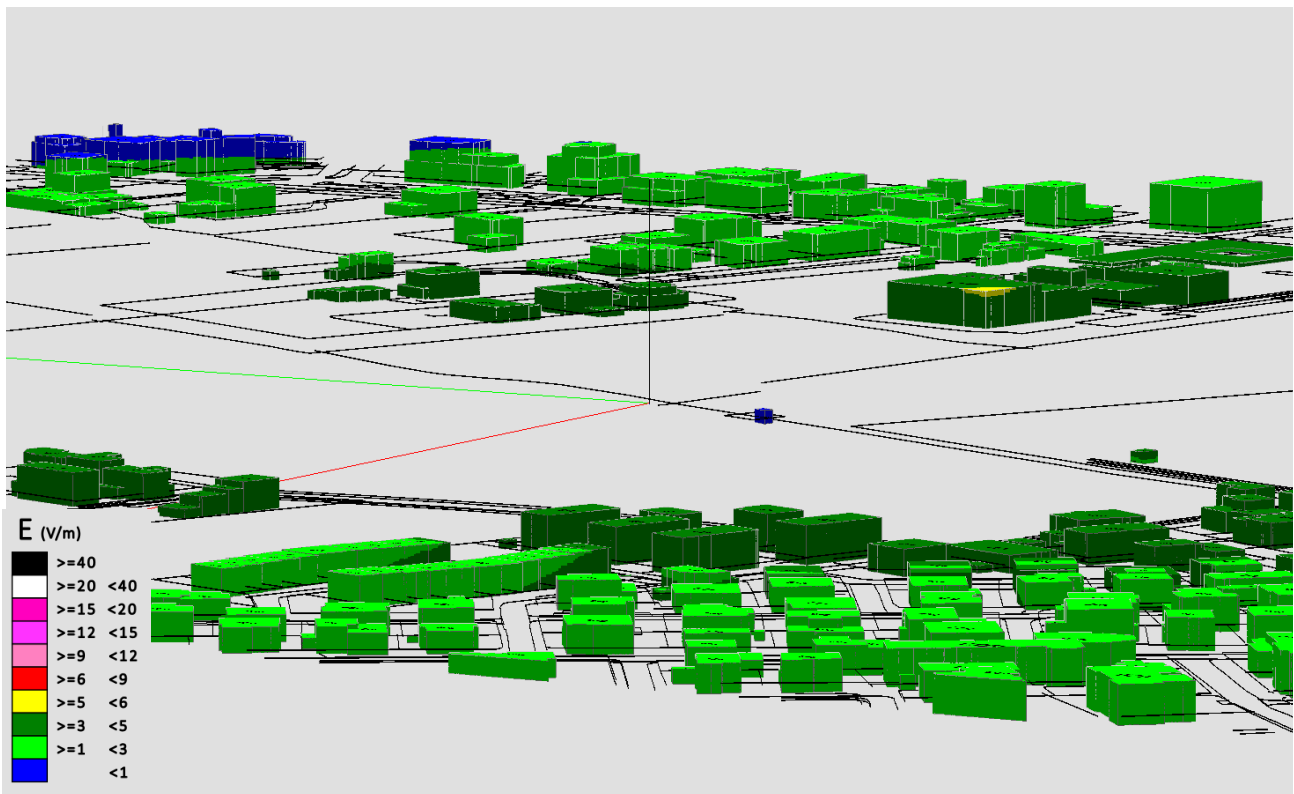
Fig. 10 Impatto elettromagnetico - Zona Via dei Carabinieri - Vista laterale senza solido
