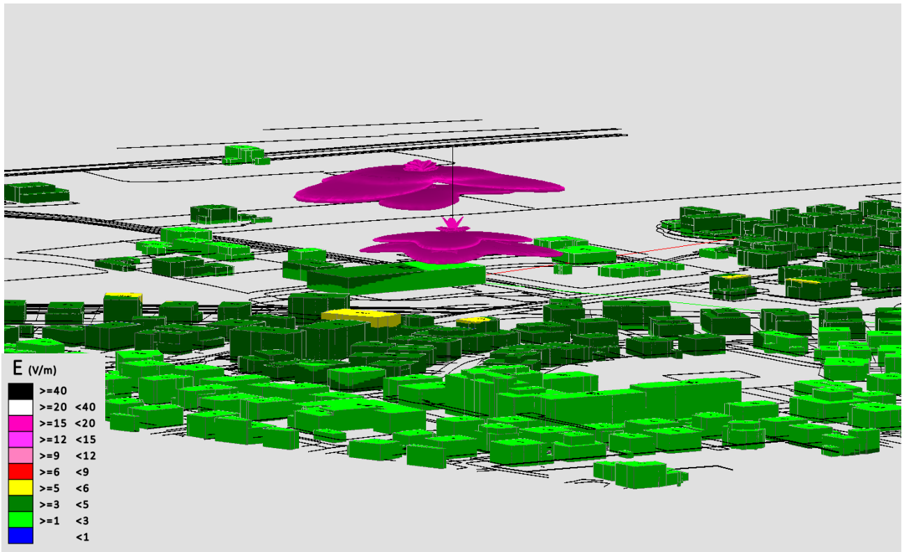
Fig. 4 Impatto elettromagnetico - Zona Rotatoria Via dei Colli Via Battisti Via Montesanto - Vista laterale
