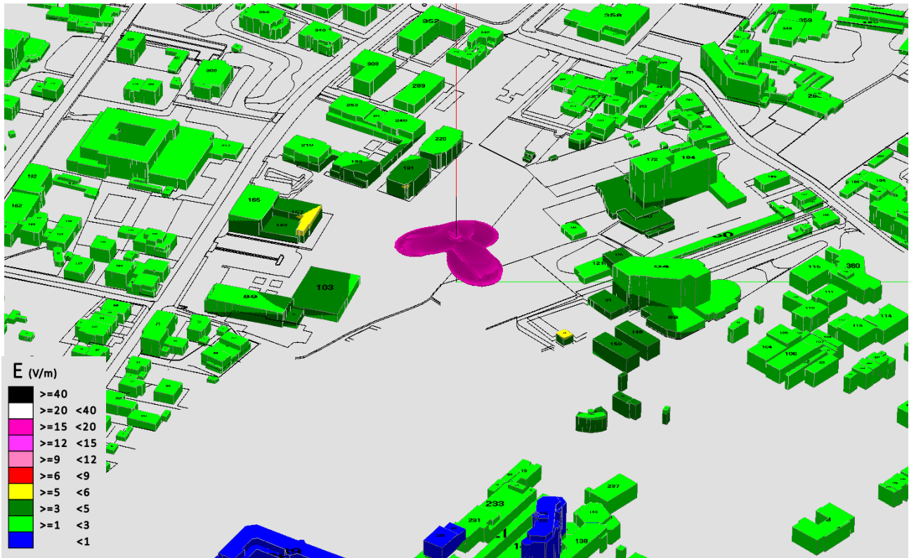
Fig. 47 Impatto elettromagnetico - Zona Via Busonera - 0° N
