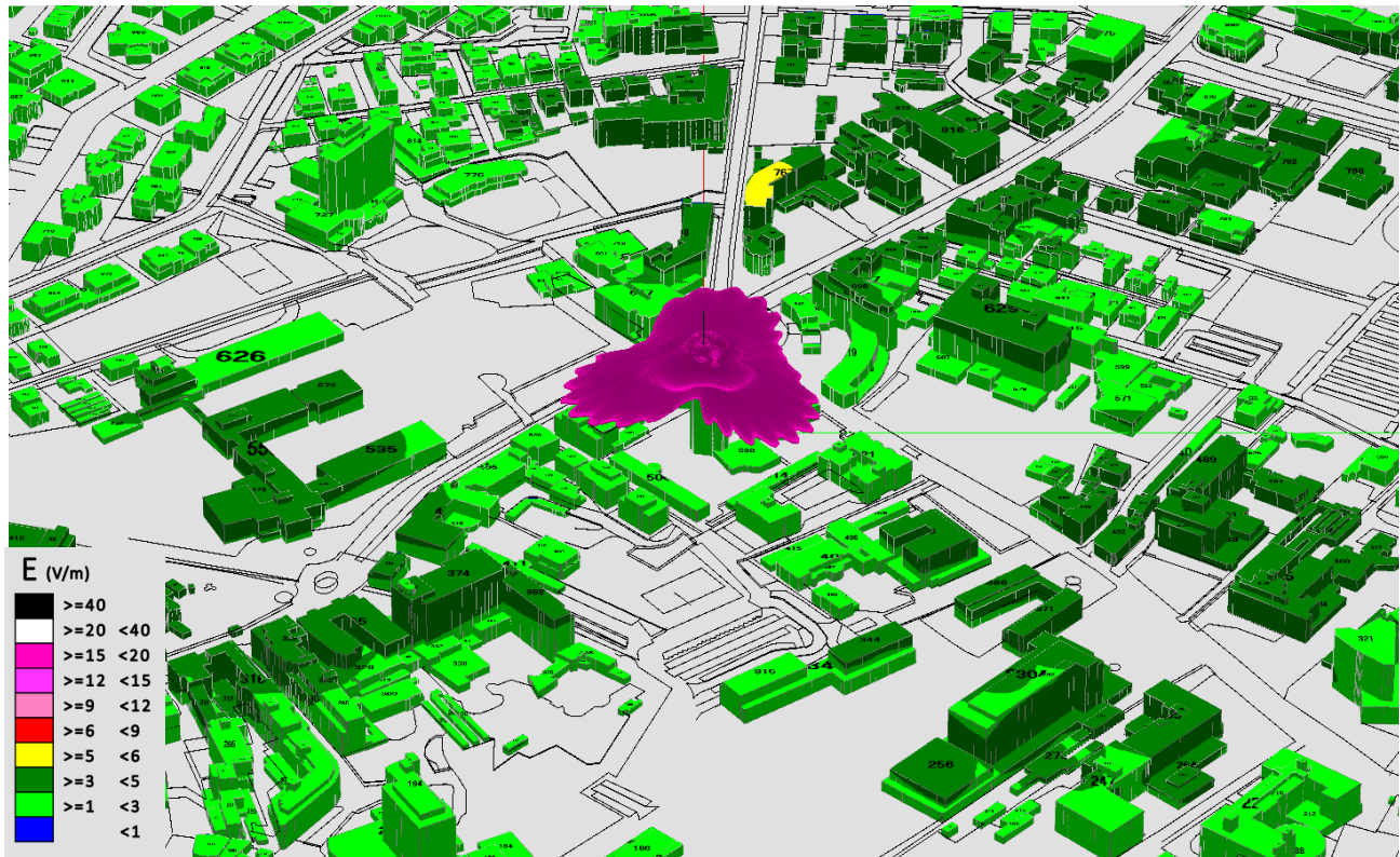
Fig. 22 Impatto elettromagnetico - Zona Abano Centro - 0° N
