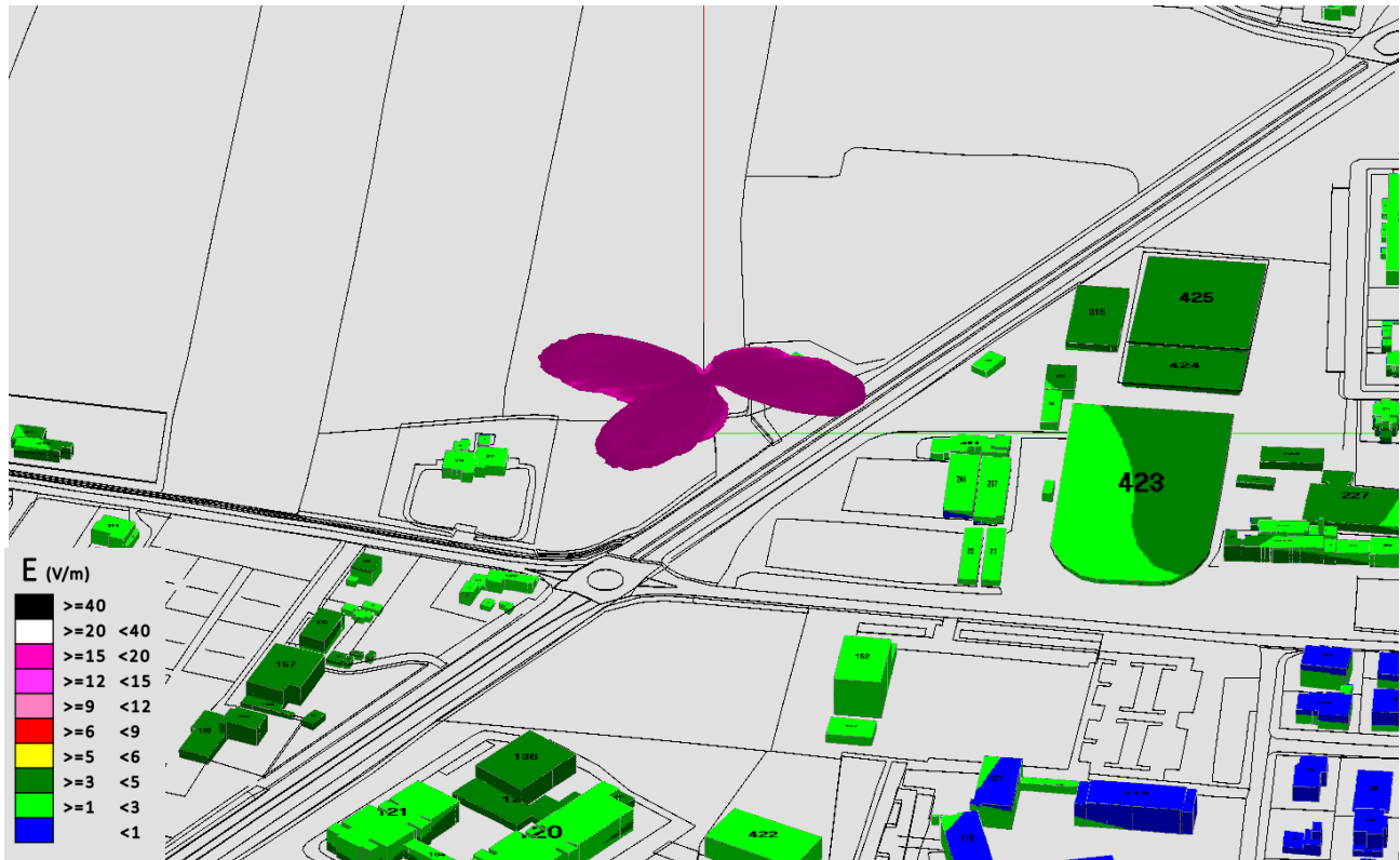
Fig. 12 Impatto elettromagnetico - Zona Area Orti Sociali - 0° N
