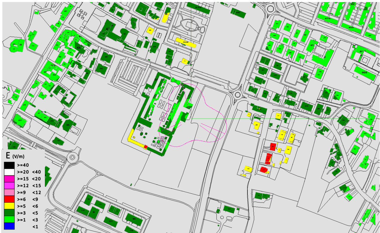
Fig. 18 Impatto elettromagnetico - Zona Cimitero Via T. Livio - Vista dall'alto senza solido
