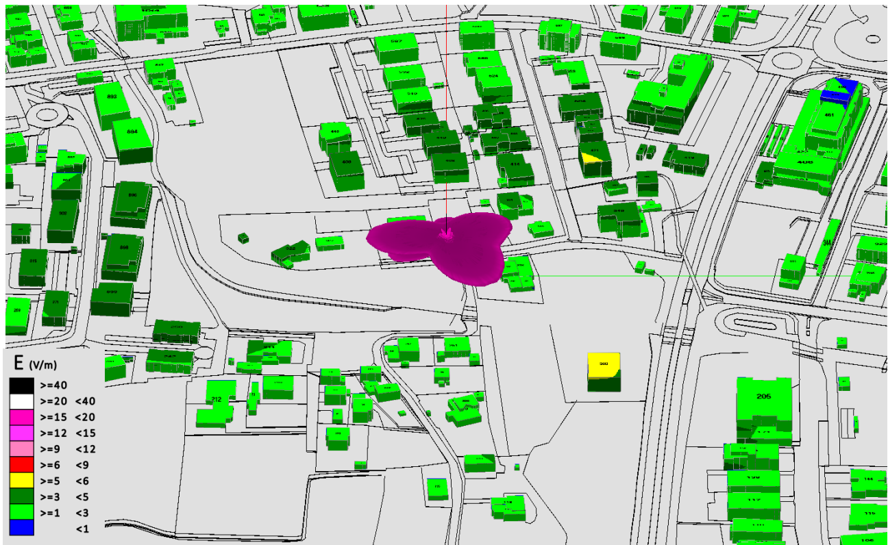
Fig. 32 Impatto elettromagnetico - Zona Via Monte Croce - 0° N
