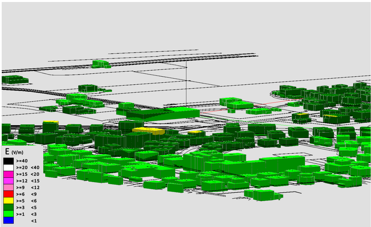
Fig. 5 Impatto elettr. - Zona Rotatoria Via dei Colli Via Battisti Via Montesanto - Vista laterale senza solido
