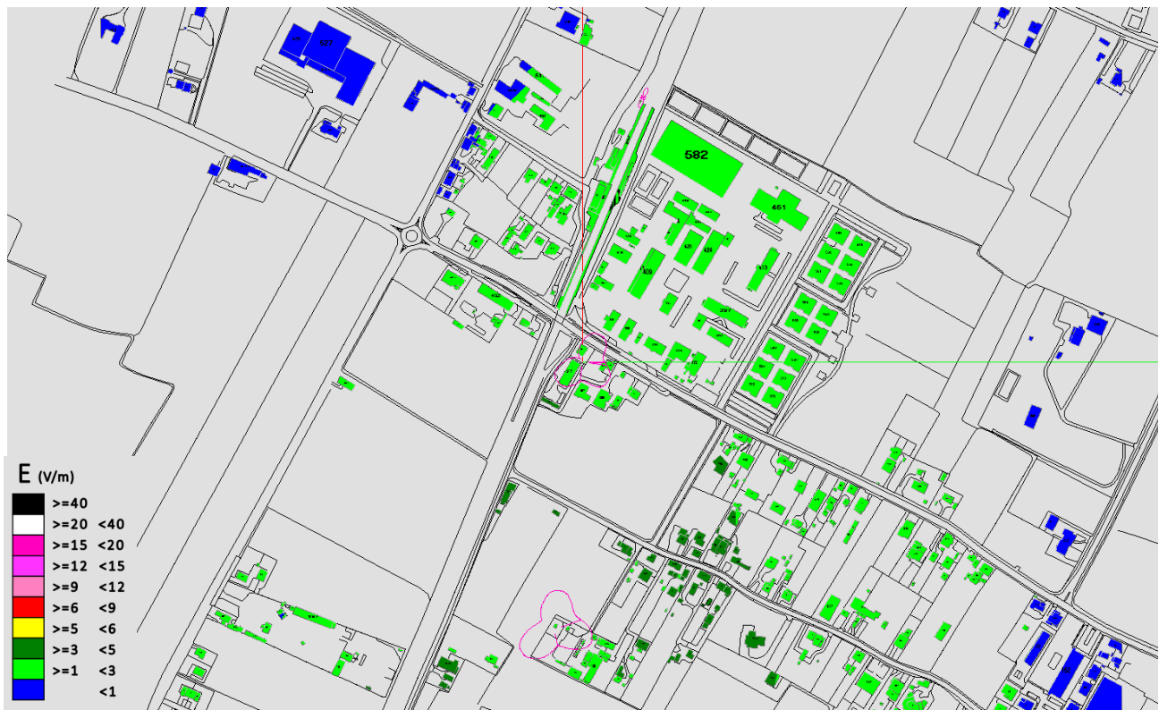
Fig. 38 Impatto elettr. - Zona Via Stazione Via Podrecca Via Levante Ferrovia - Vista dall'alto senza solido
