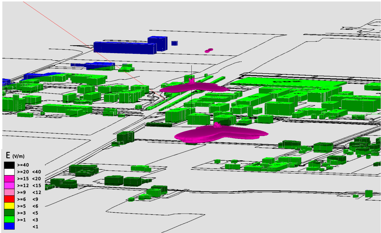
Fig. 39 Impatto elettromagnetico - Zona Via Stazione Via Podrecca Via Levante Ferrovia - Vista laterale
