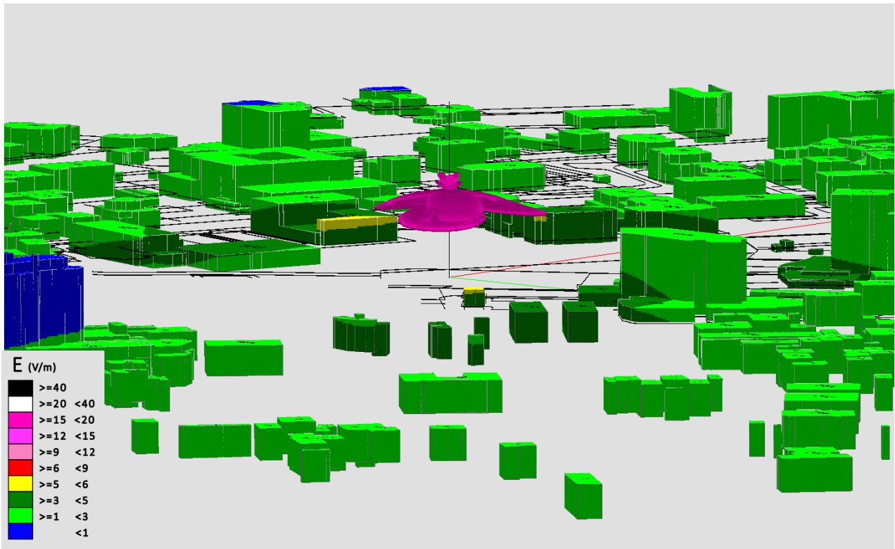
Fig. 49 Impatto elettromagnetico - Zona Via Busonera - Vista laterale
