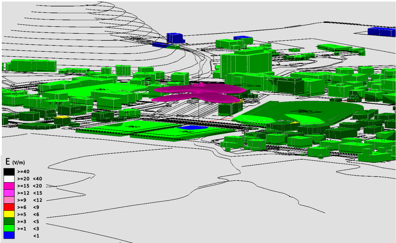
Fig. 29 Impatto elettromagnetico - Zona Stadio Comunale - Vista laterale
