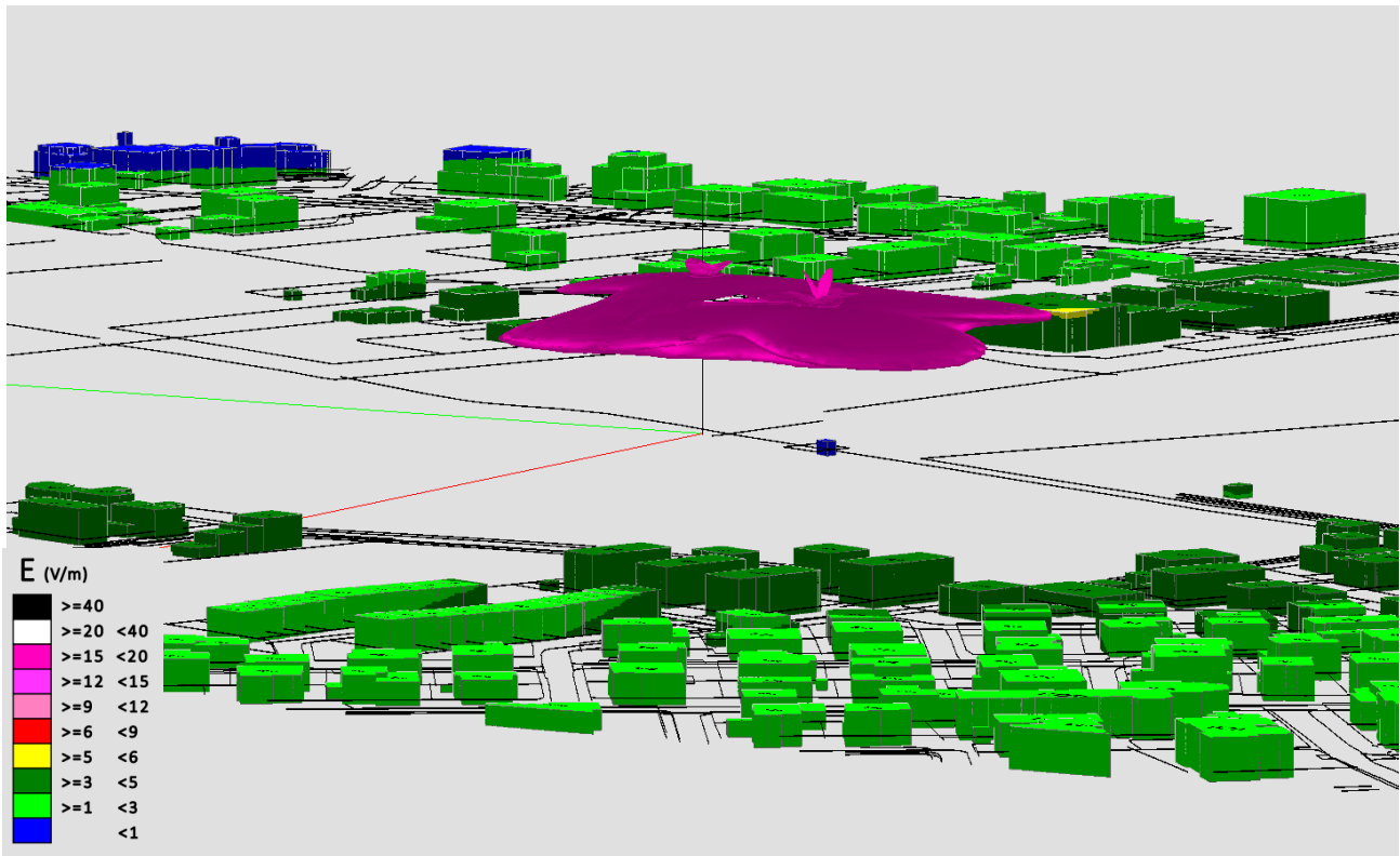
Fig. 9 Impatto elettromagnetico - Zona Via dei Carabinieri - Vista laterale
