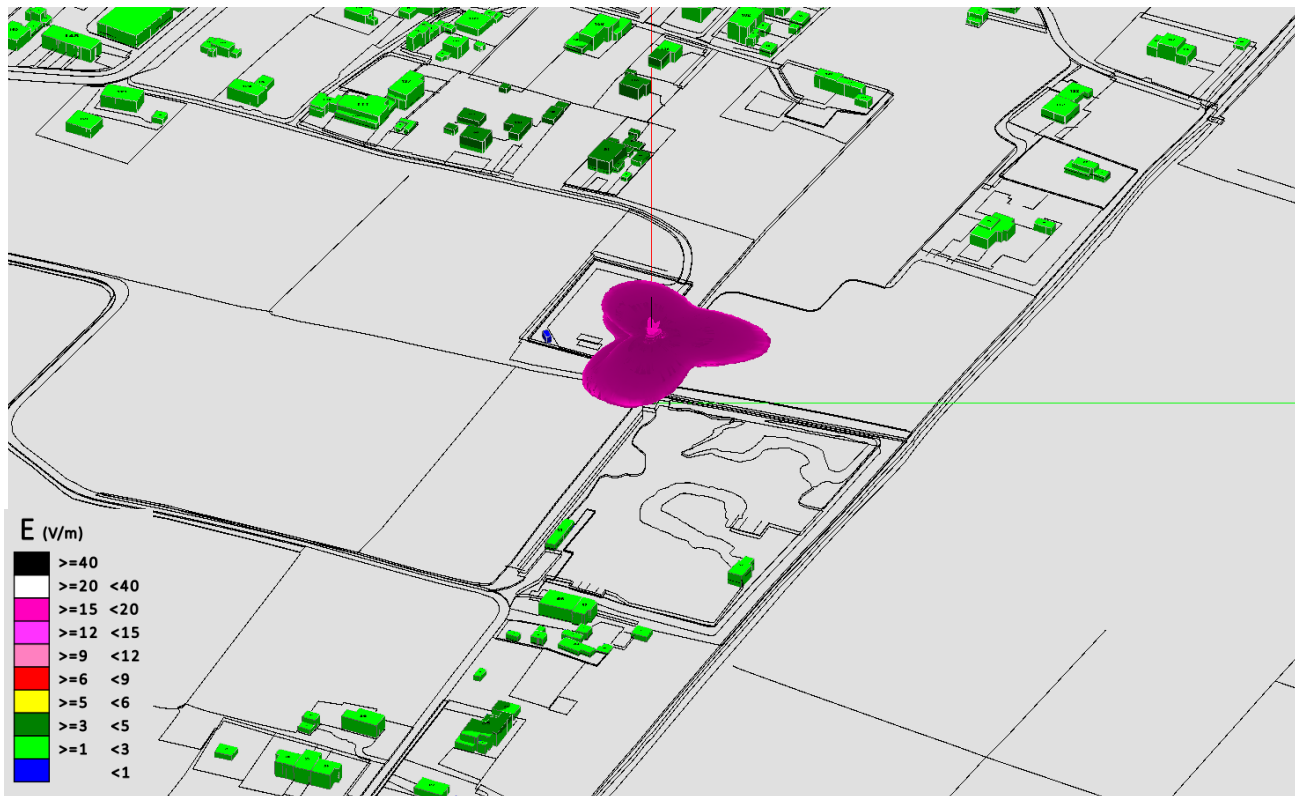
Fig. 52 Impatto elettromagnetico - Zona Giarre Via S. Giustina - 0° N
