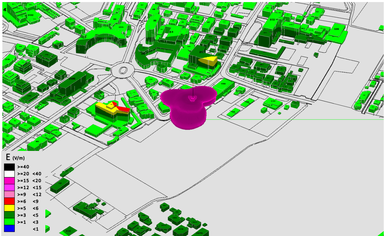
Fig. 42 Impatto elettromagnetico - Zona Via Pacinotti - Parcheggio - 0° N
