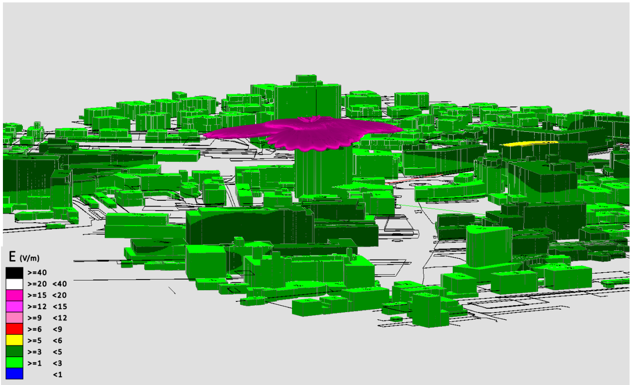
Fig. 24 Impatto elettromagnetico - Zona Abano Centro - Vista laterale
