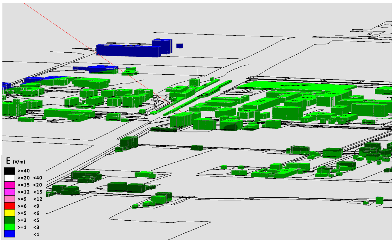
Fig. 40 Impatto elettr. - Zona Via Stazione Via Podrecca Via Levante Ferrovia - Vista laterale senza solido
