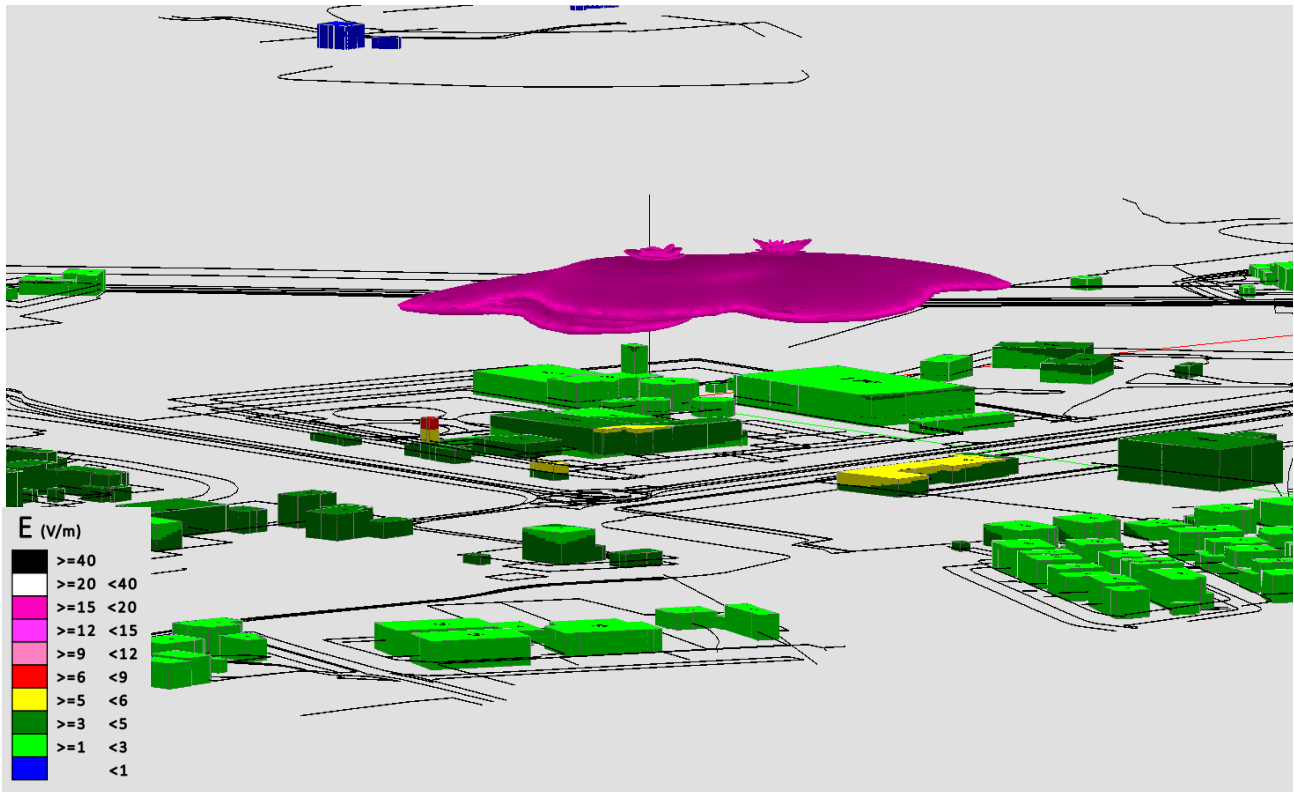
Fig. 59 Impatto elettromagnetico - Zona Depuratore Comunale - Vista laterale
