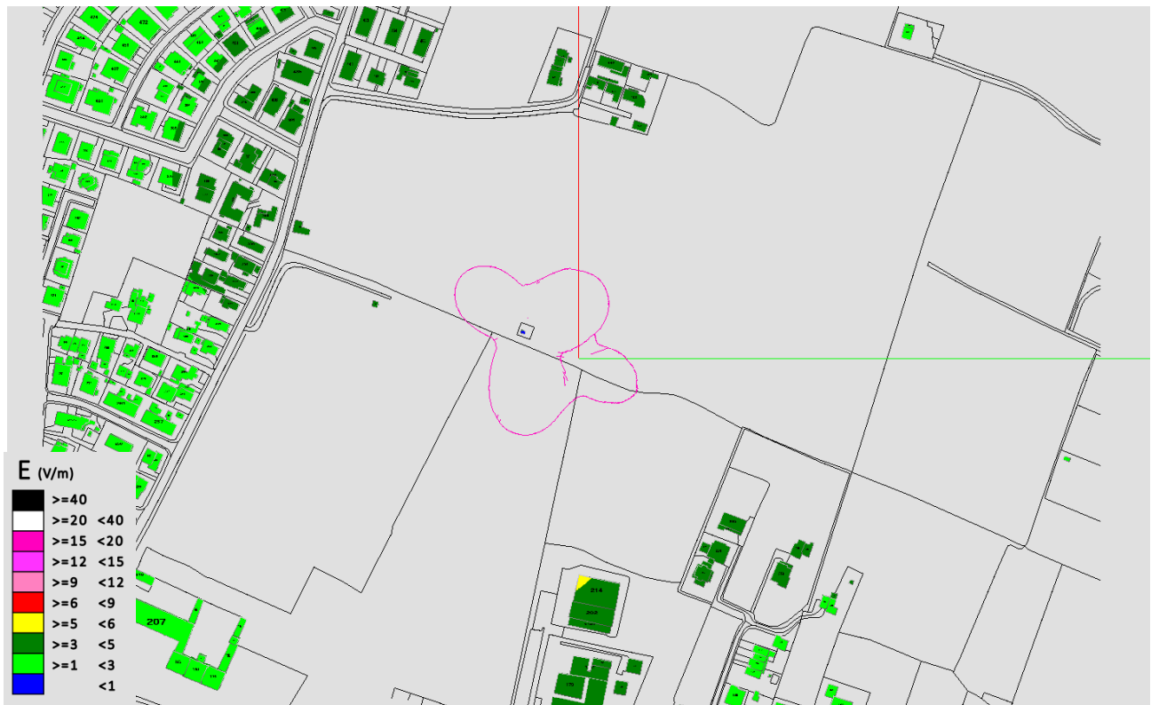
Fig. 8 Impatto elettromagnetico - Zona Via dei Carabinieri - Vista dall'alto senza solido
