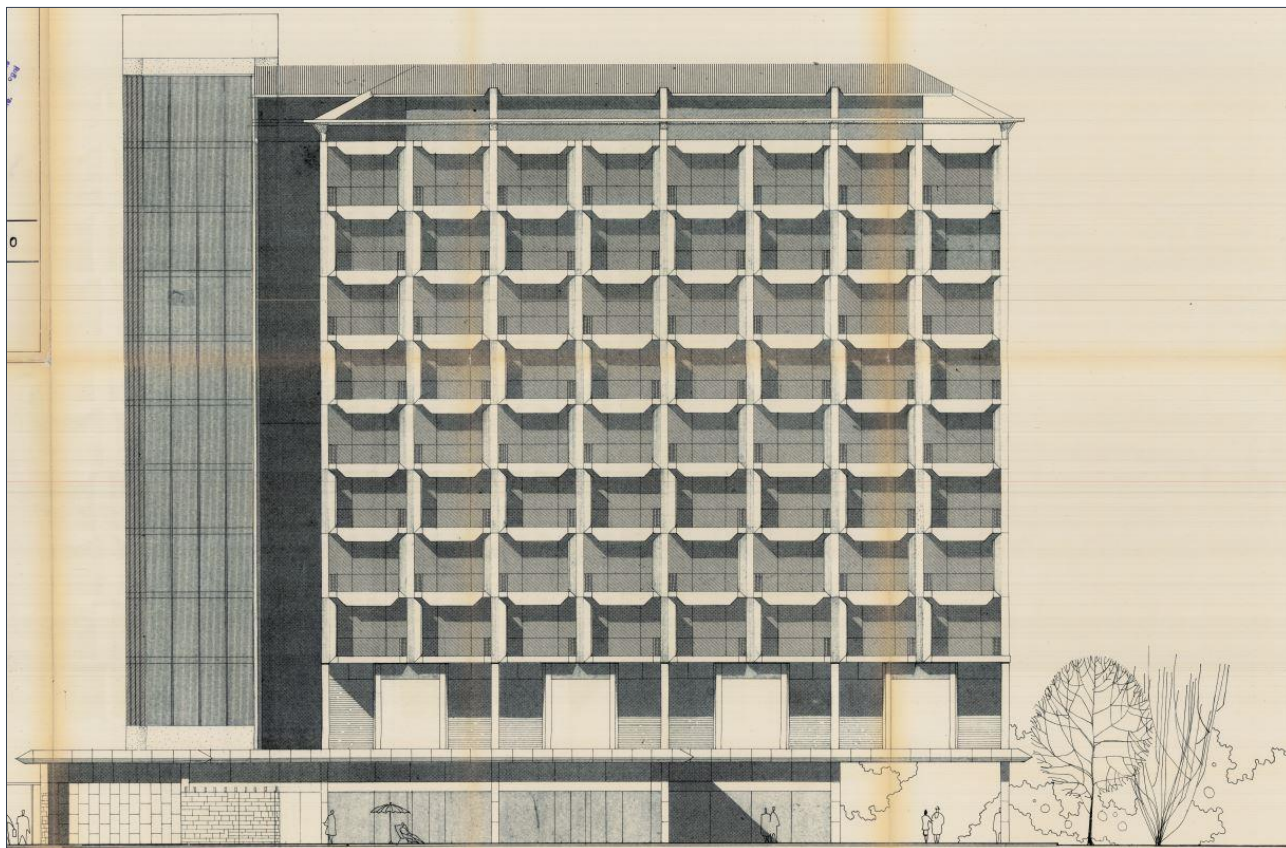
Estratto tavola prospetto est Hotel Centrale
