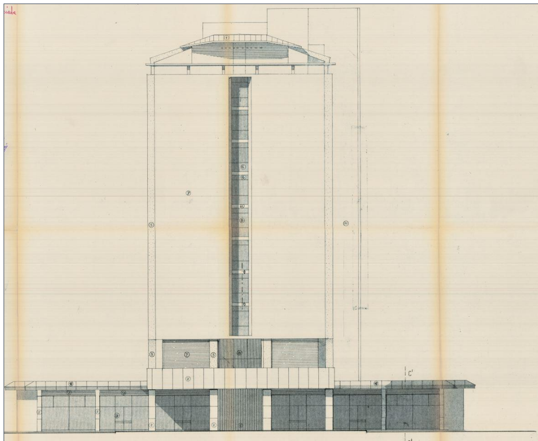
Estratto tavola prospetto sud Hotel Centrale
