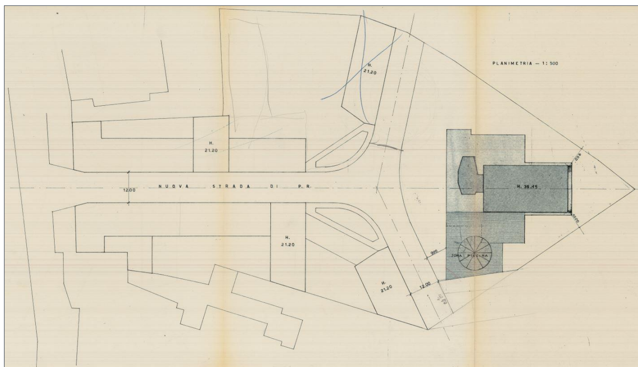
Estratto tavola planimetria Hotel Centrale
